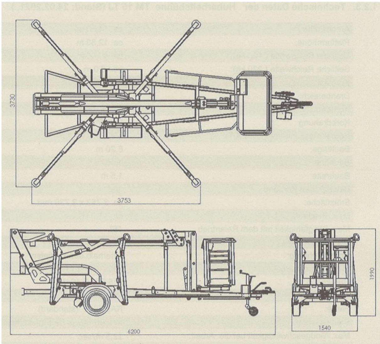
1. Abb.: Abmessungen der Arbeitsbühne TM 15 TJ
